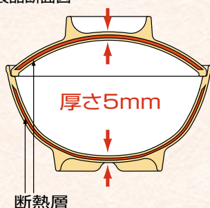
■製品断面図
